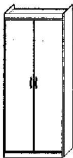
skriňa šatníková výška: 1900mm šírka: 800mm hĺbka: 500mm
